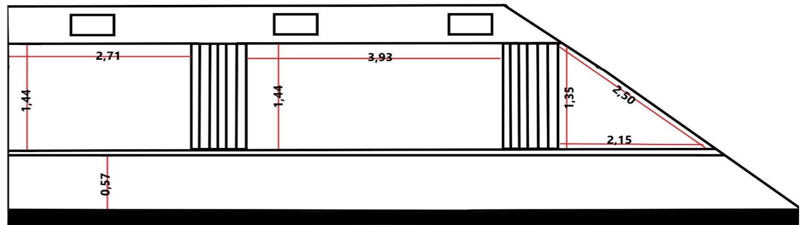
Alzado Lateral Planta Baja
