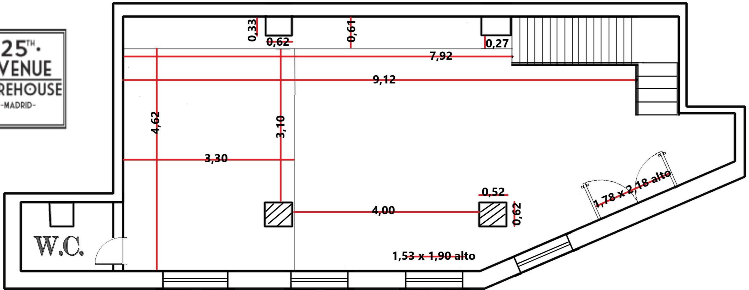
Frontal Planta Baja
